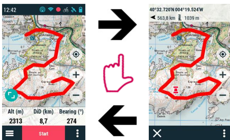
MODE 'DONNÉES'
